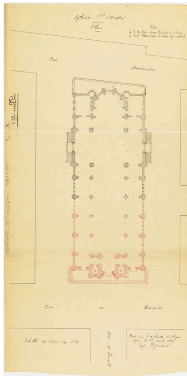
Plan d'achèvement de l'église Saint-André (1897) (Arch. mun. Lyon, 954 WP 58, Paul Desjardins, dessin).
