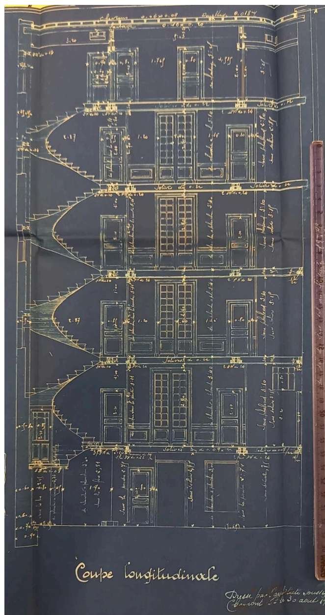
Coupe longitudinale, 43 avenue d'Italie
