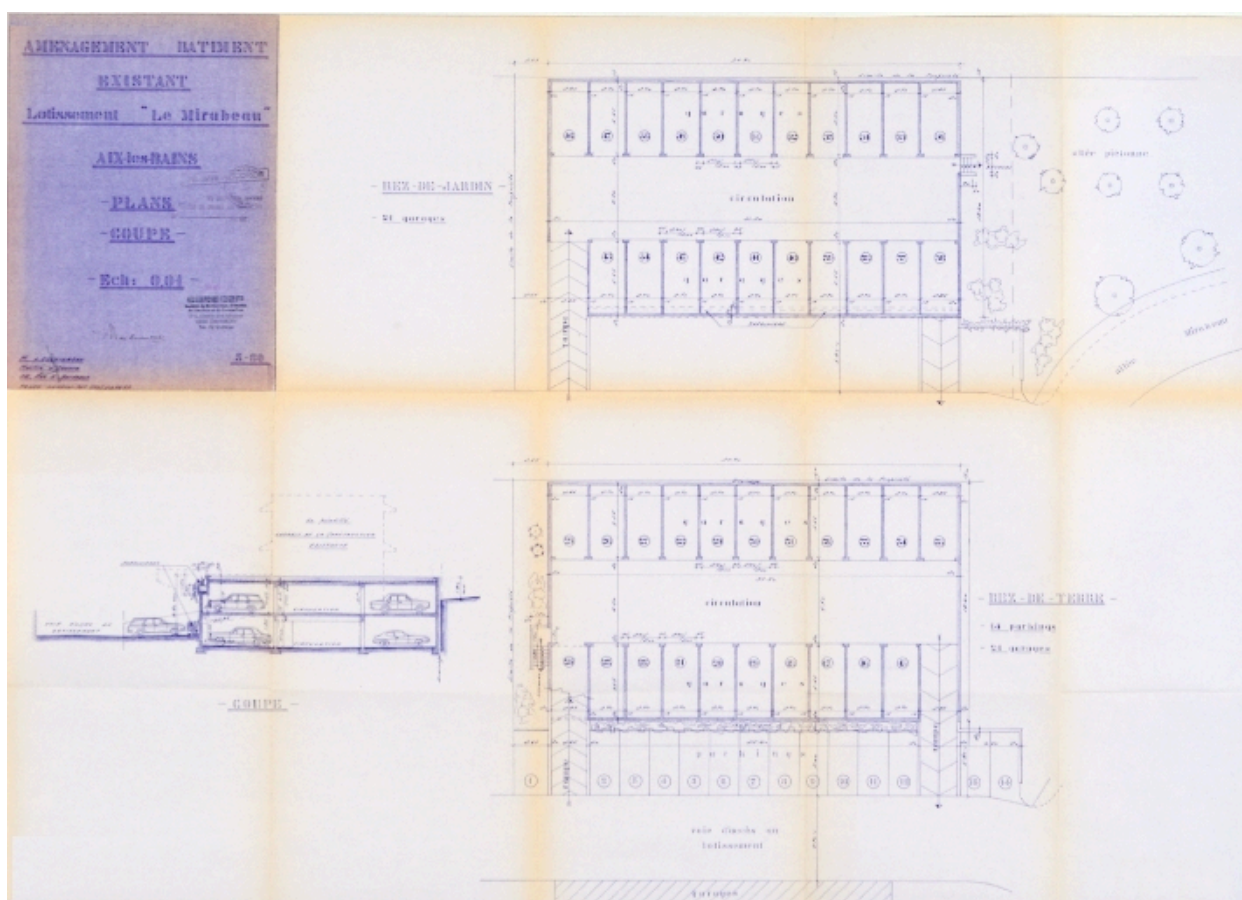
Coupe et plans des garages, 1979
