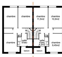
Plan de l'étage
