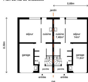
Plan du rez-de-chaussée
