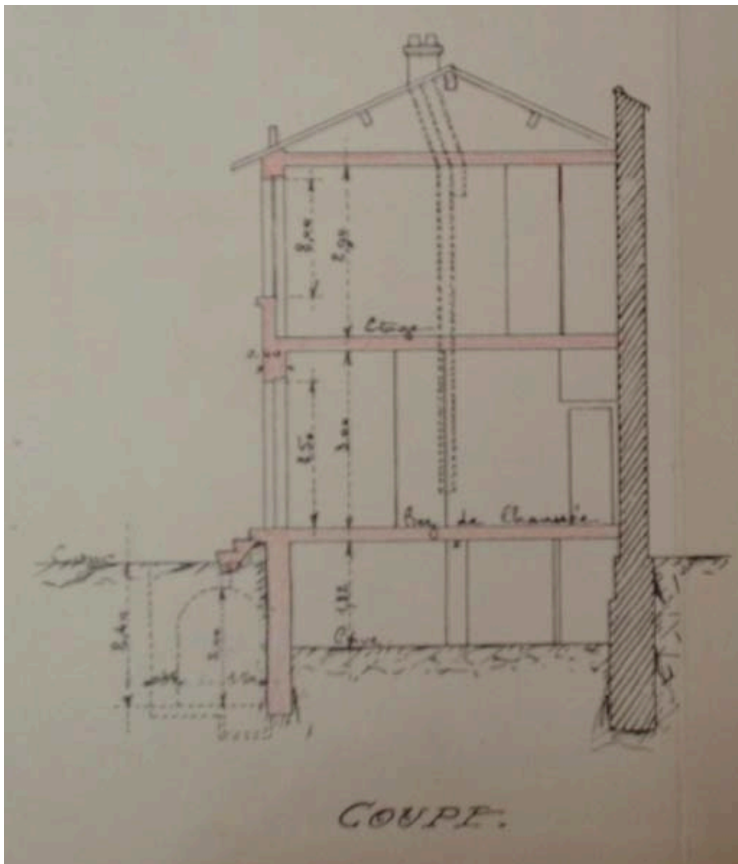
Ets Brossette ; construction de 6 logements ; coupe (1925)
