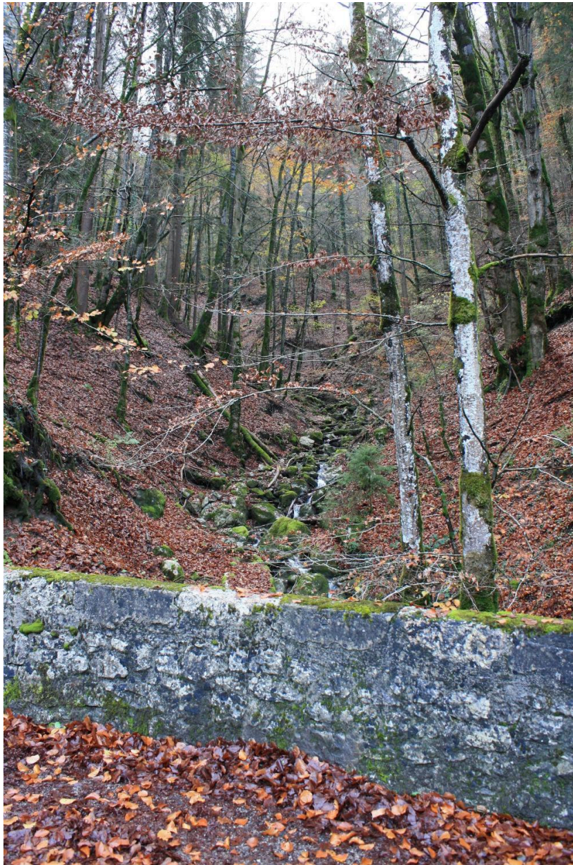
Pont de Trélachaud, contexte et garde corps amont
