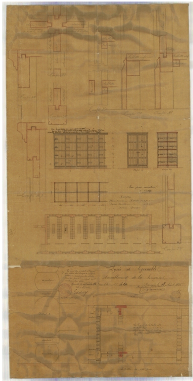
Plan. Détail d'ameublement de la lingerie. 18 août 1886.
