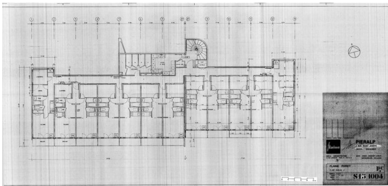
Plan du 1er étage. M.B. A architectes, SCPA Jossa, Chiquet, Loehr, Michahelles, Vallejos architectes, 2 décembre 1986 (AC Arâches-la-Frasse)
