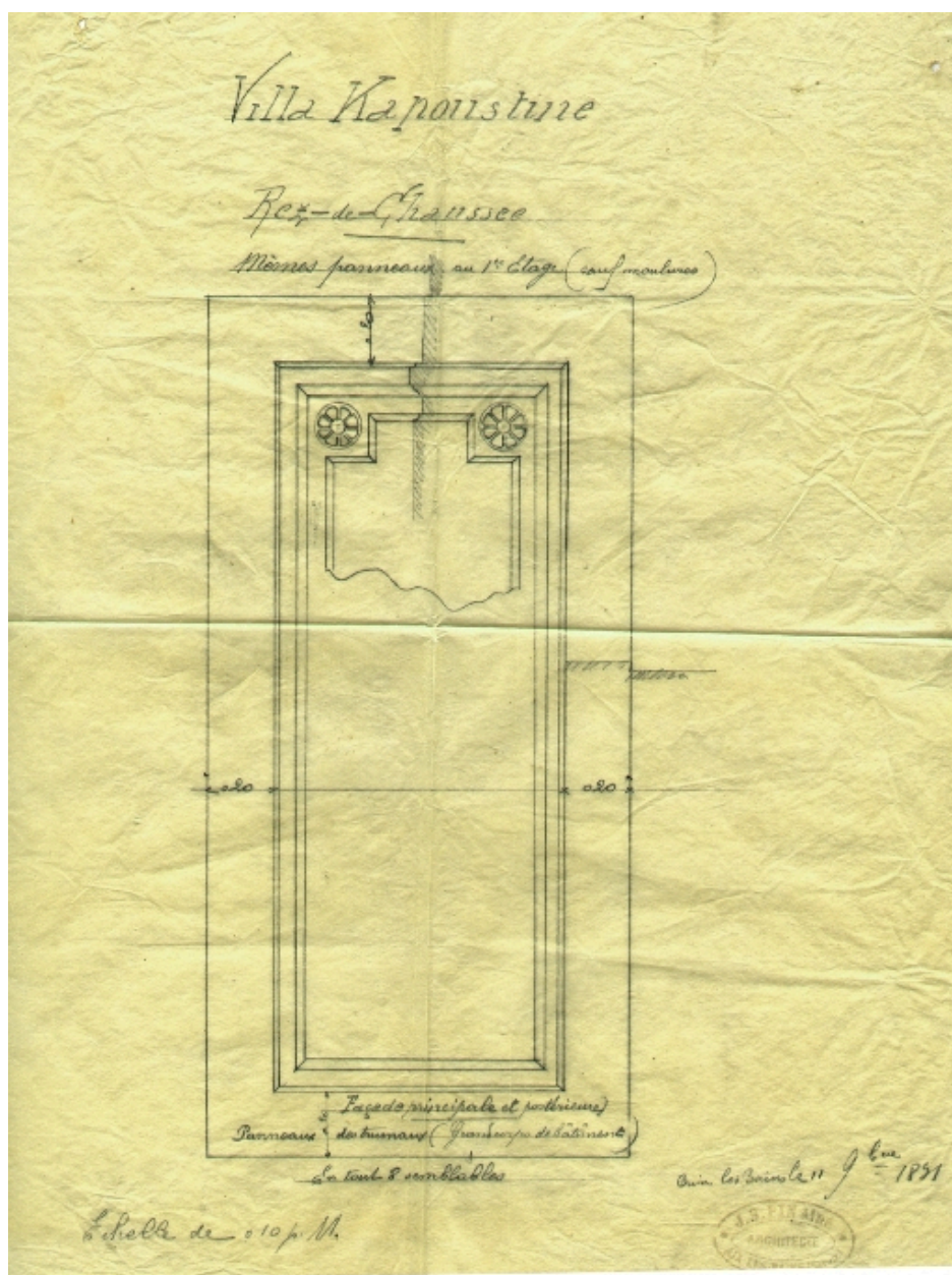
Dessin d'un trumeau de façade
