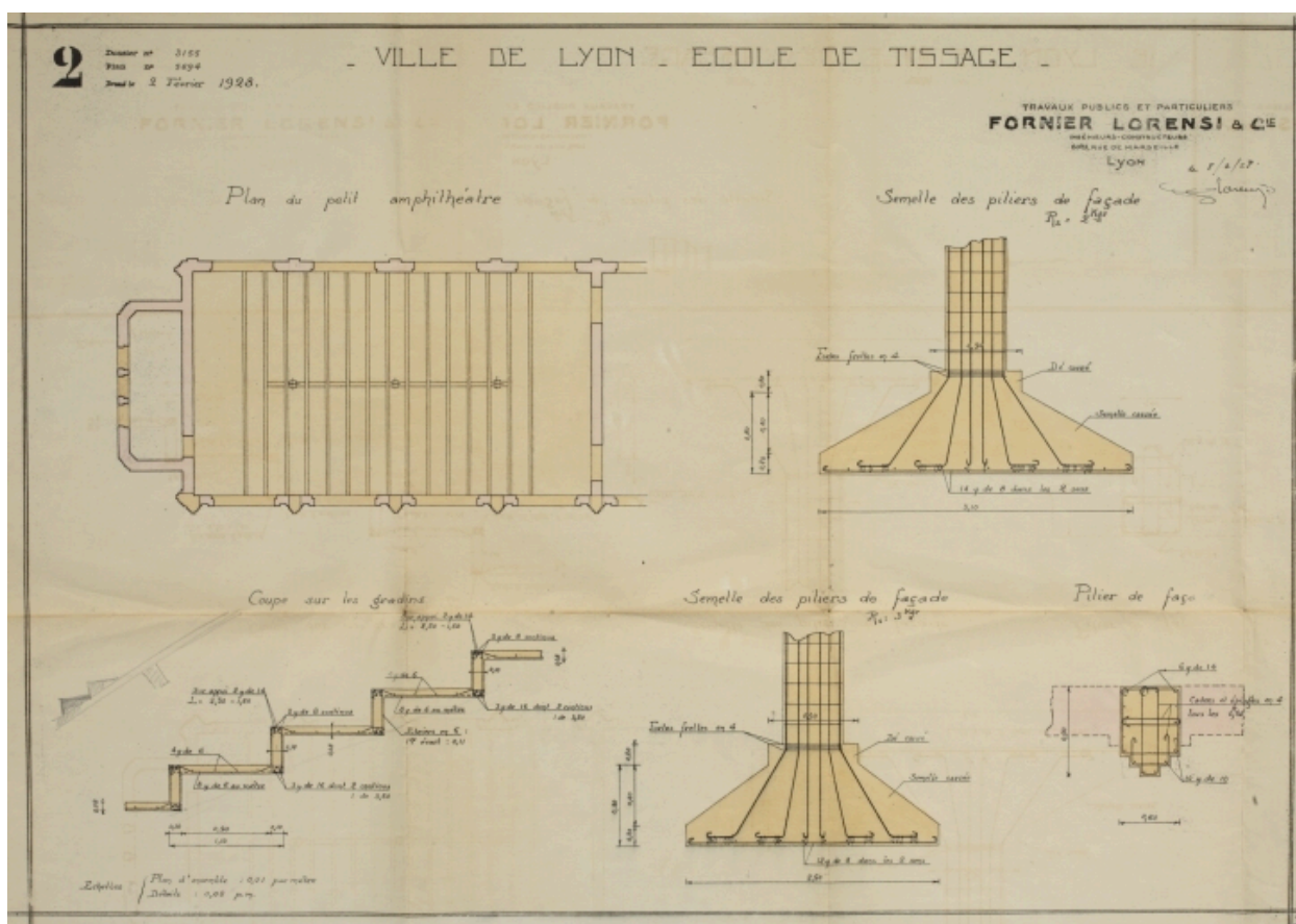
Ecole de tissage, Plan du petit amphithéâtre. 2 février 1928. Fournier Lorensi & Cie, ingénieurs constructeurs. (AC Lyon. 511 WP 002)
