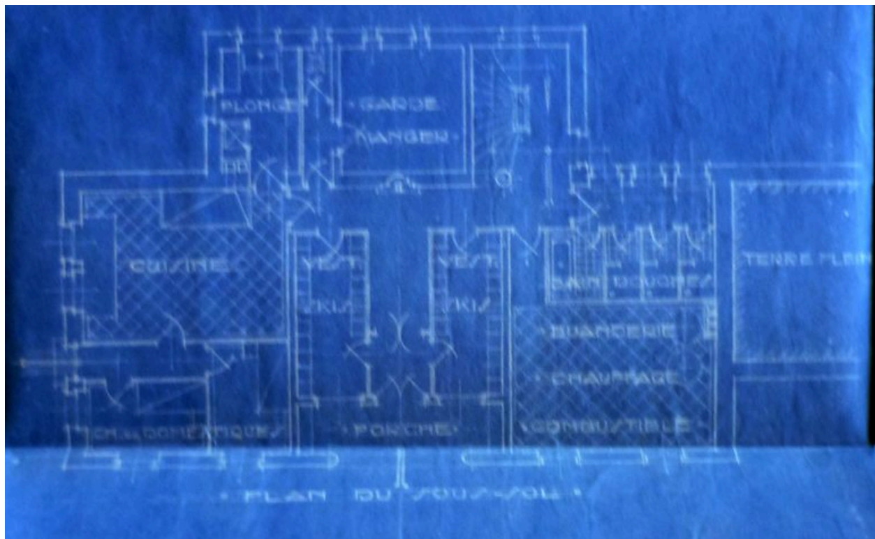
Plan du sous-sol. Henry Jacques le Même, [1926] (AD Haute-Savoie. 142J 439)
