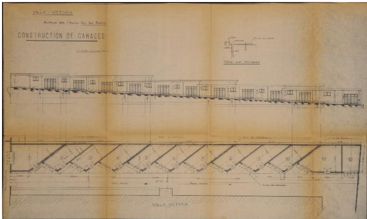
Construction de garages : plan, élévation, 1958
