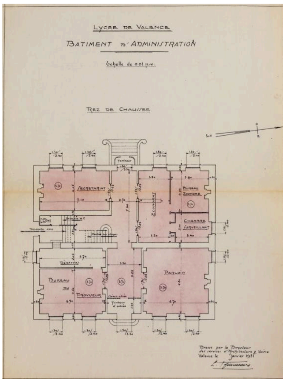
Bâtiment d'aministration. Rez-de-chaussée, 1931
