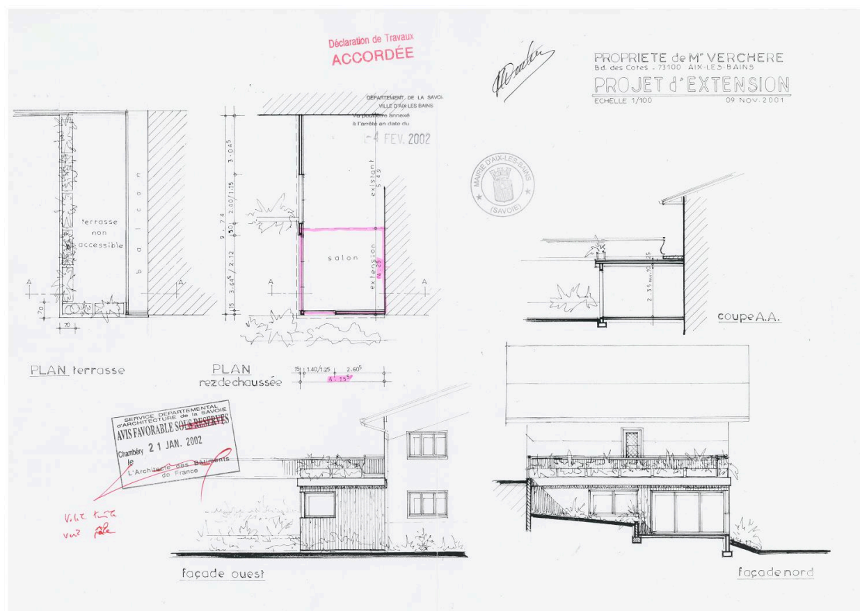
Projet d'extension : plans, façades et coupe, 2001
