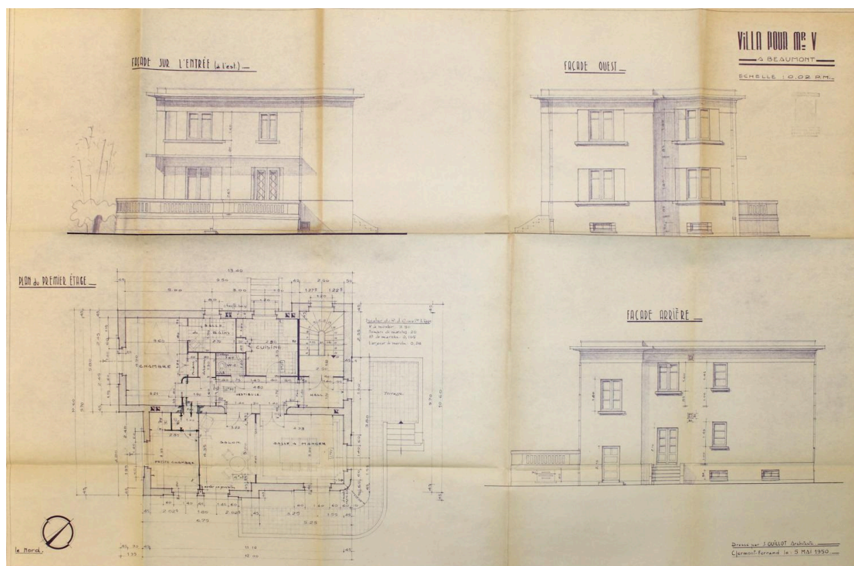
Beaumont, la maison V., plan du premier étage, façades latérales et arrière, Jean Guillot architecte, 5 mai 1950 (archives départementales du Puy-de-Dôme).
