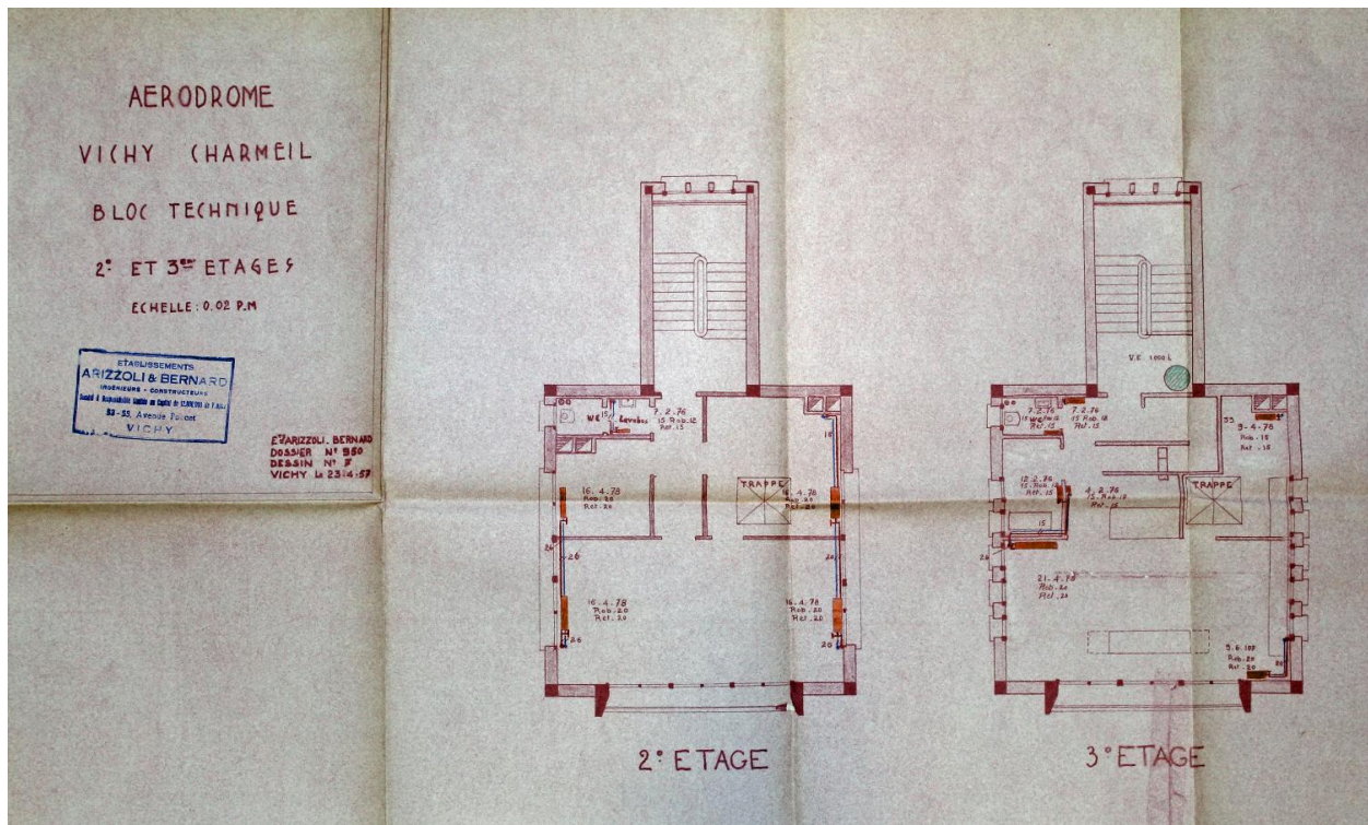
Plan des 2e et 3e étages du bloc technique de l'aérogare de Vichy-Charmeil, 1957, Service technique des bases aériennes (Archives municipales de Vichy).
