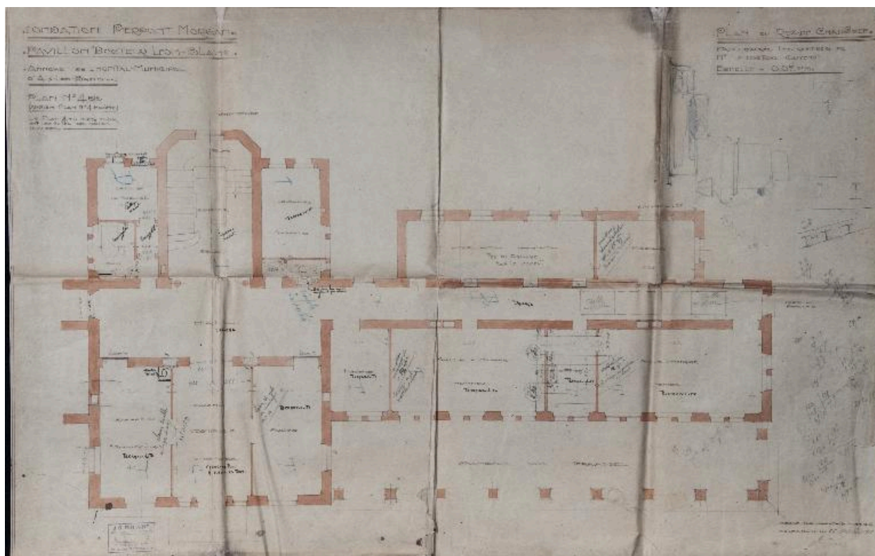
Aile est, 1911 : plan du 1er étage
