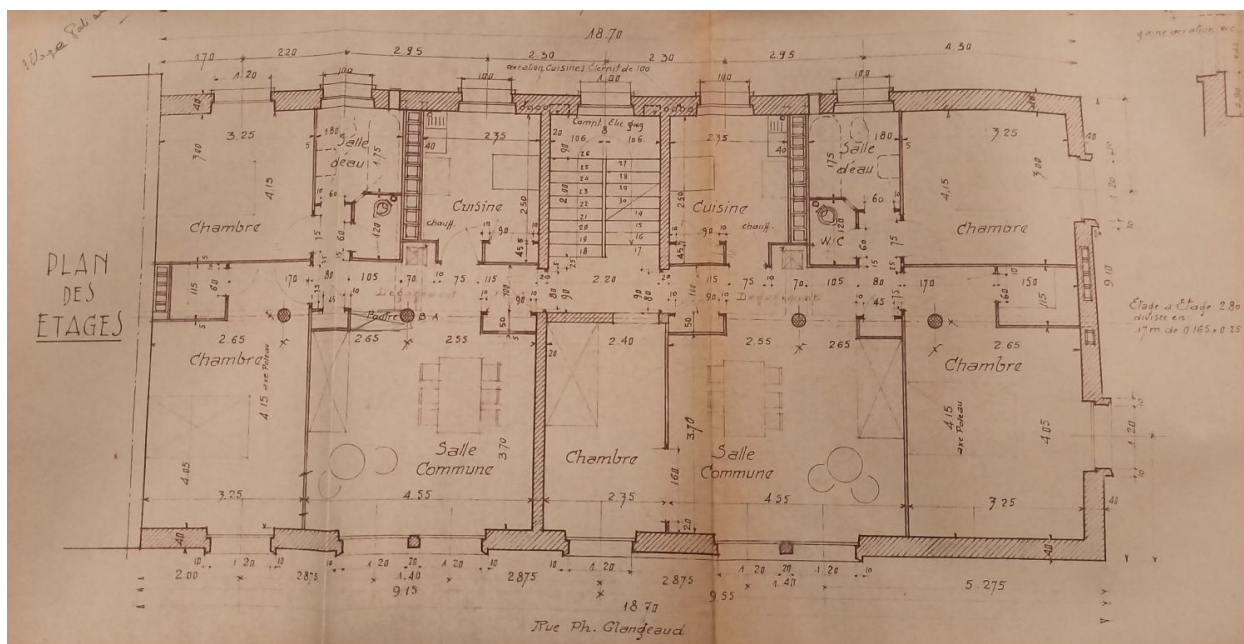
Plan des étages
