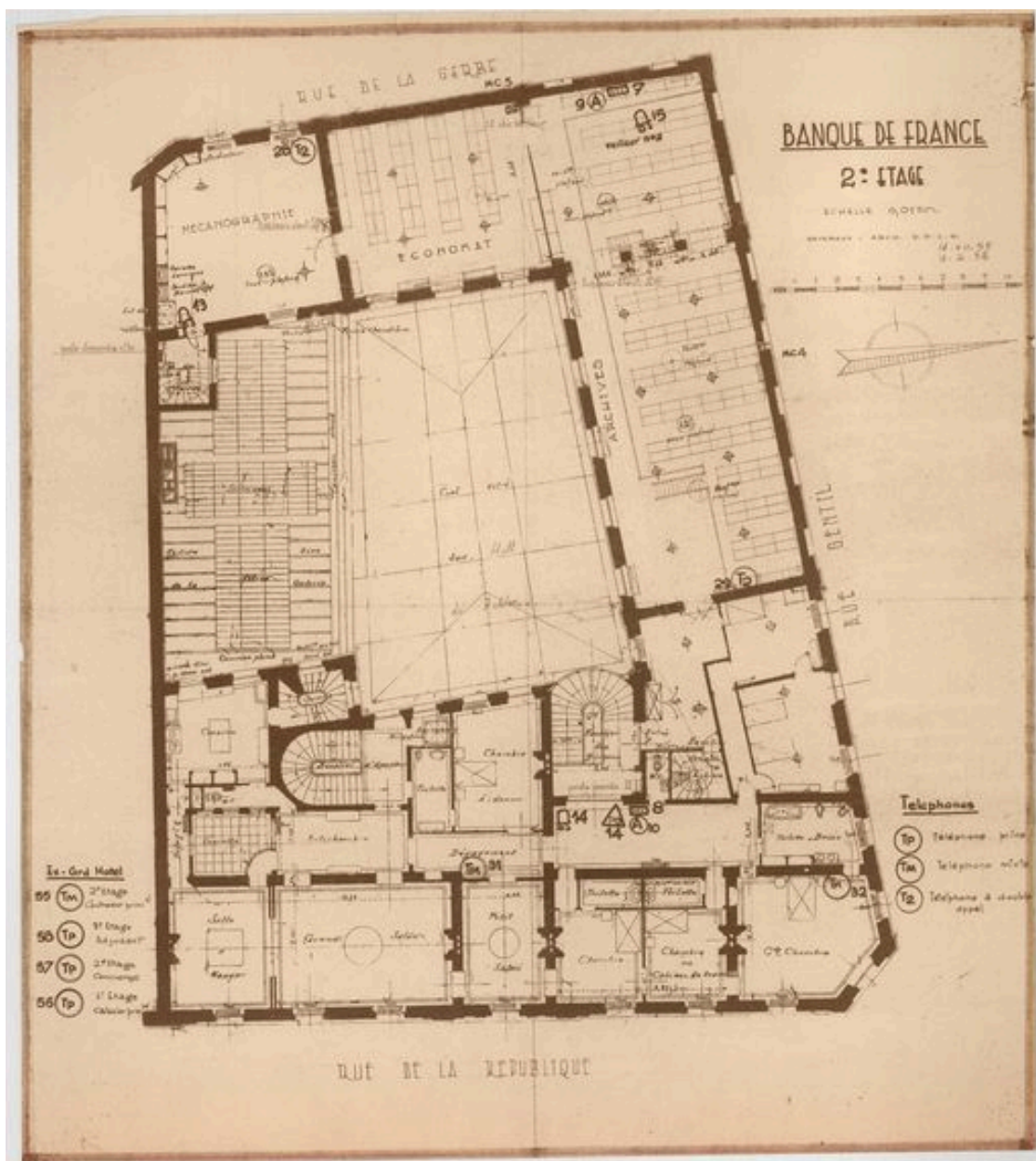
Plan du second étage avec l'exhaussement de la verrière (1955) (Banque de France, PHAR, non coté, Gabriel Deveraux, tirage d'architecte).
