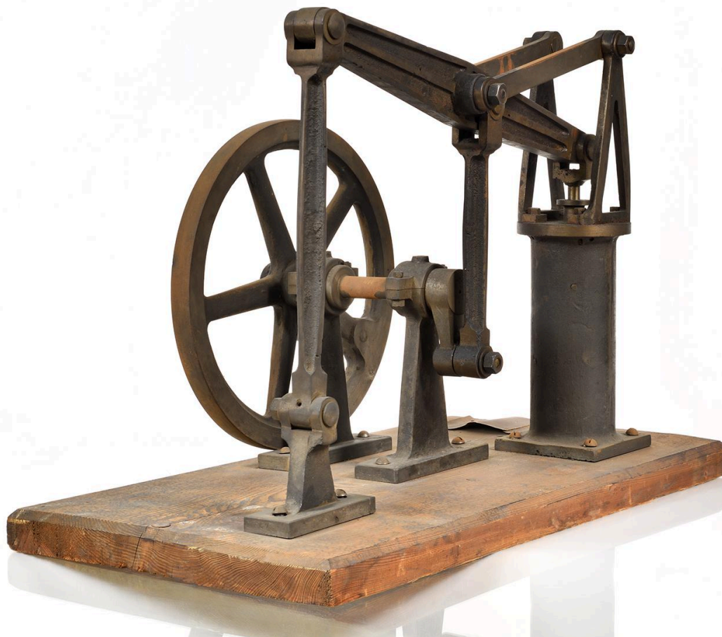
Modèle de pompe, vue 2
