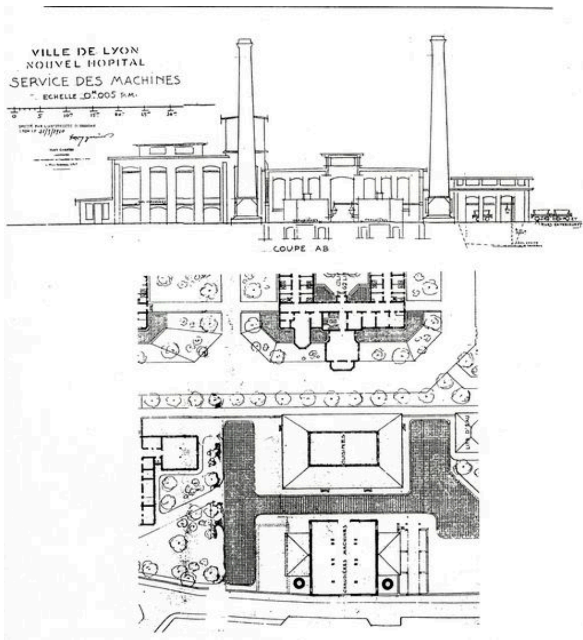
Projet de chaufferie / Tony Garnier, 31 mai 1910 (Arch. mun. Lyon)
