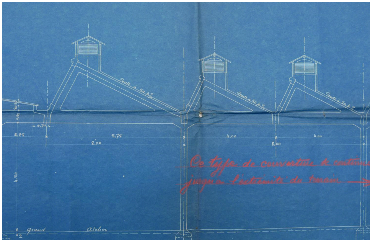
Plan usine Seguin 1917 : toiture sheds avec aérateurs (ACL 314W/581)
