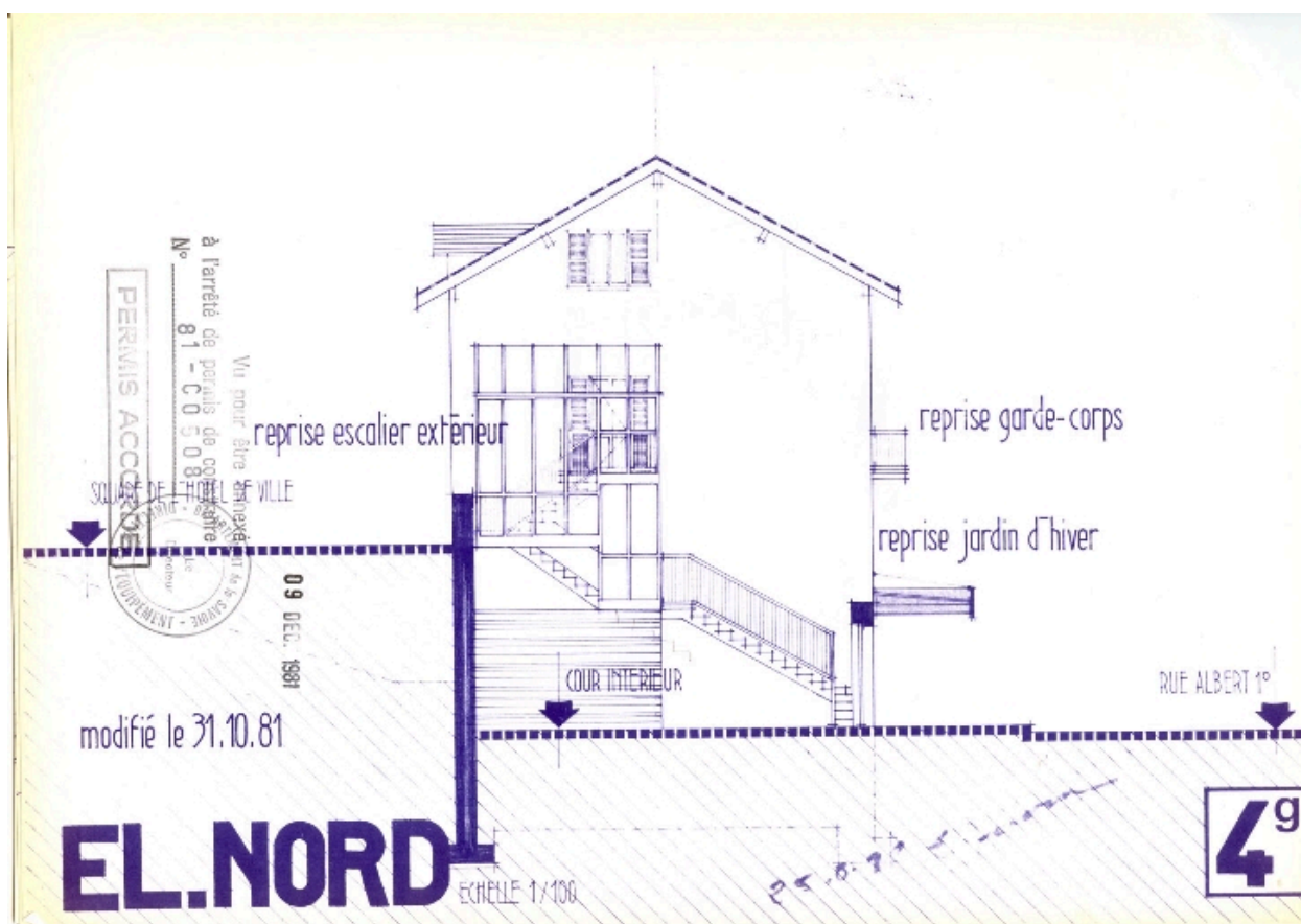
Elévation nord
