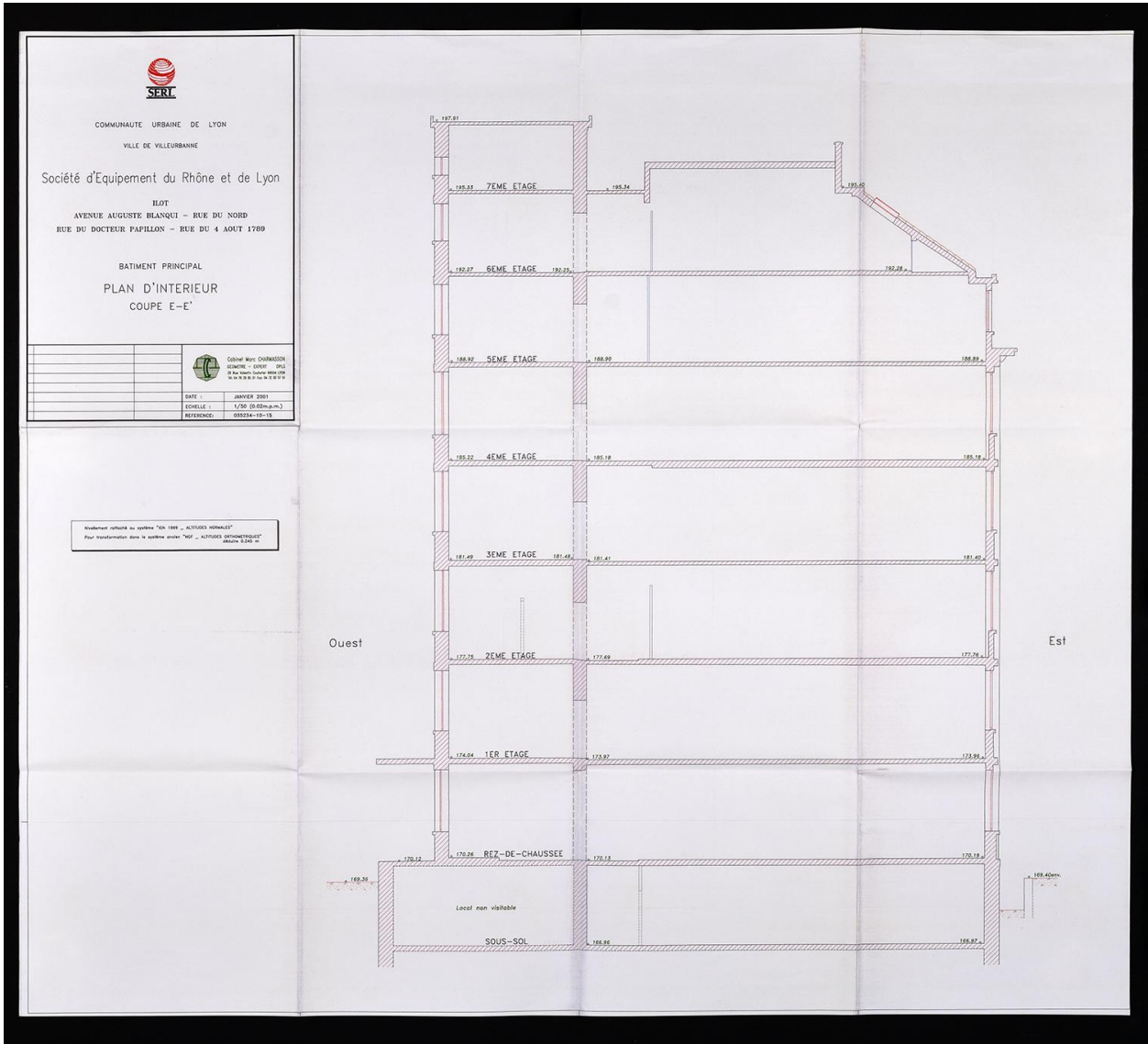
Coupe EE bâtiment principal usine Bally-Camsat
