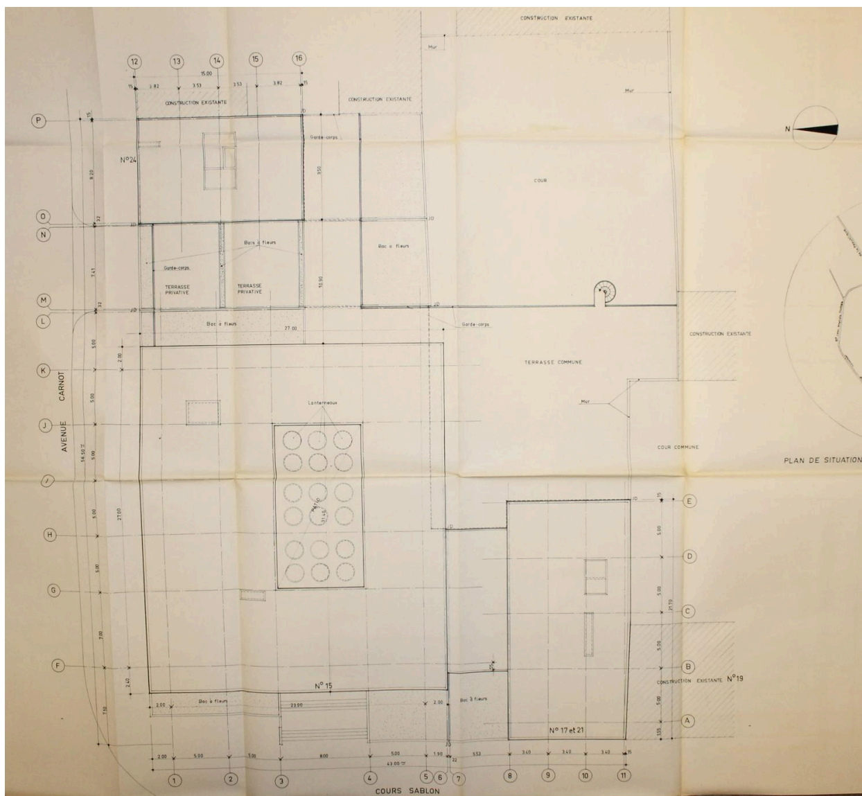
Clermont-Ferrand, succursale de la Banque de France, plan des toits-terrasses, 1971, agence ATEA Lagneau-Weil-Dimitrijevic (Archives municipales de Clermont-Ferrand, 2001 W 296).
