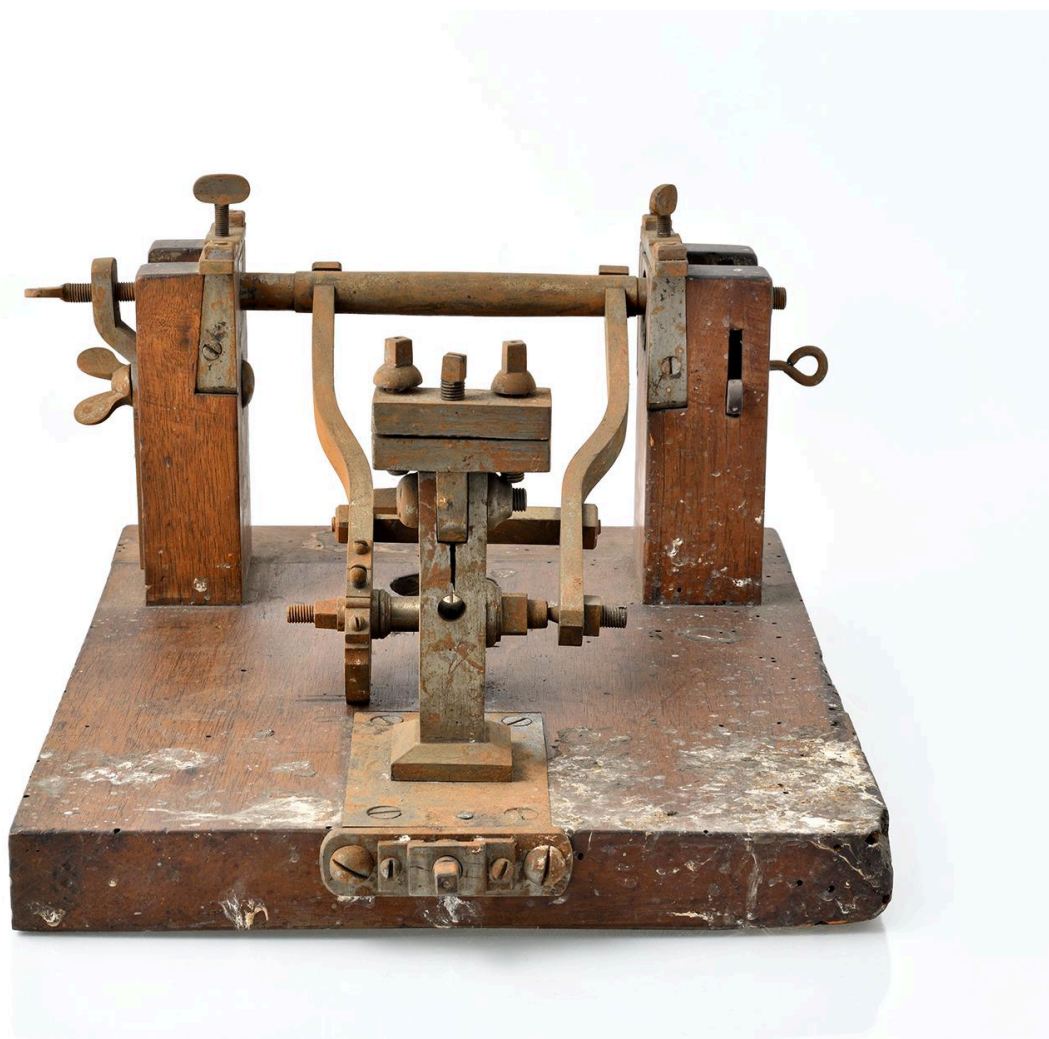
Machine à tailler les engrenages, vue 2
