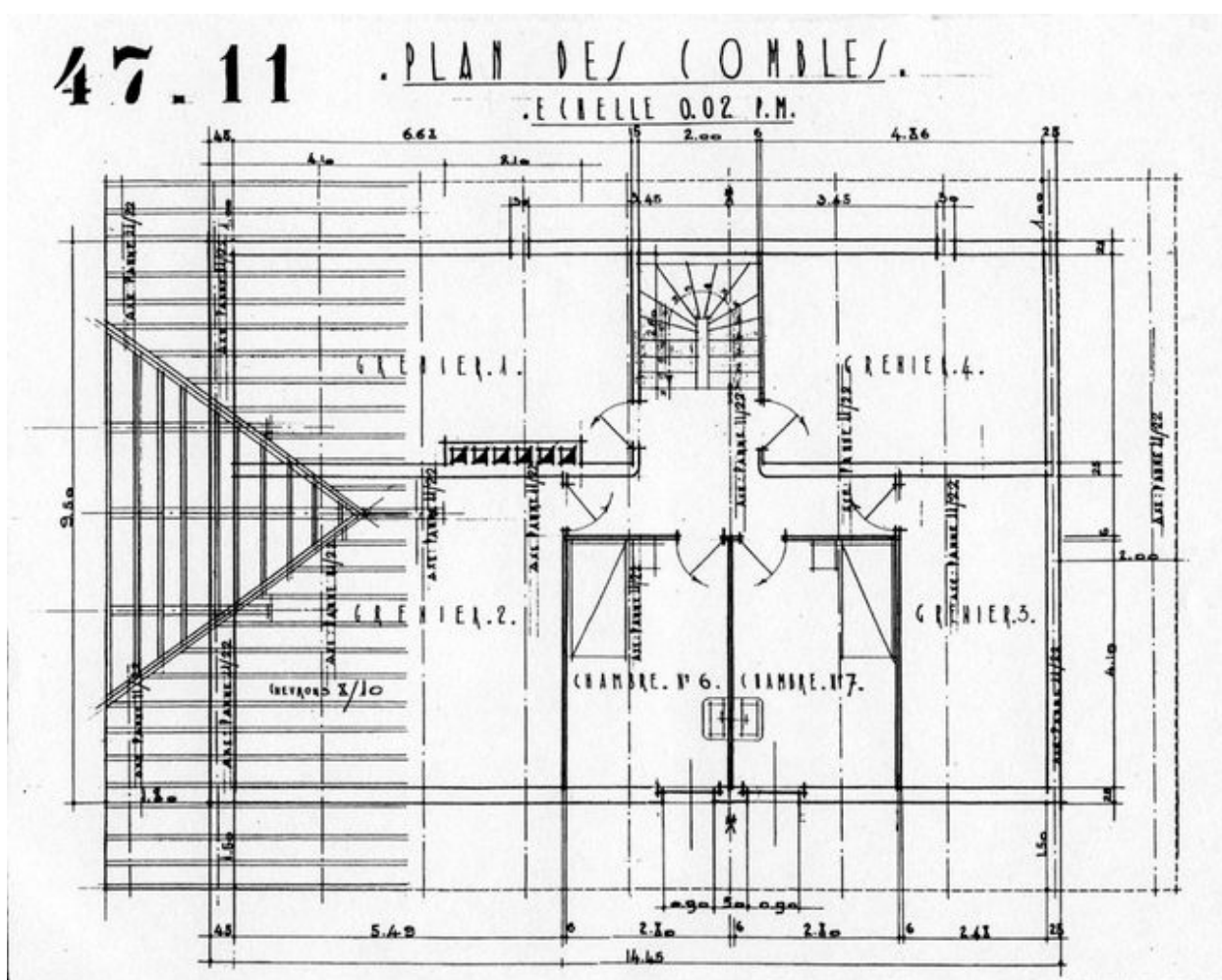
Plan des combles. Henry Jacques Le Même, [1928] (Dossier agence n° 47)
