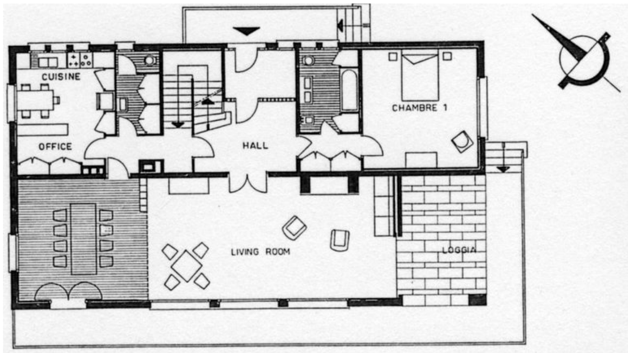
Plan du rez-de-chaussée surélevé / Henry Jacques Le Même, 1961
