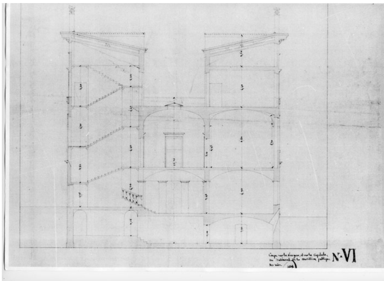
Coupe sur largeur, 1808
