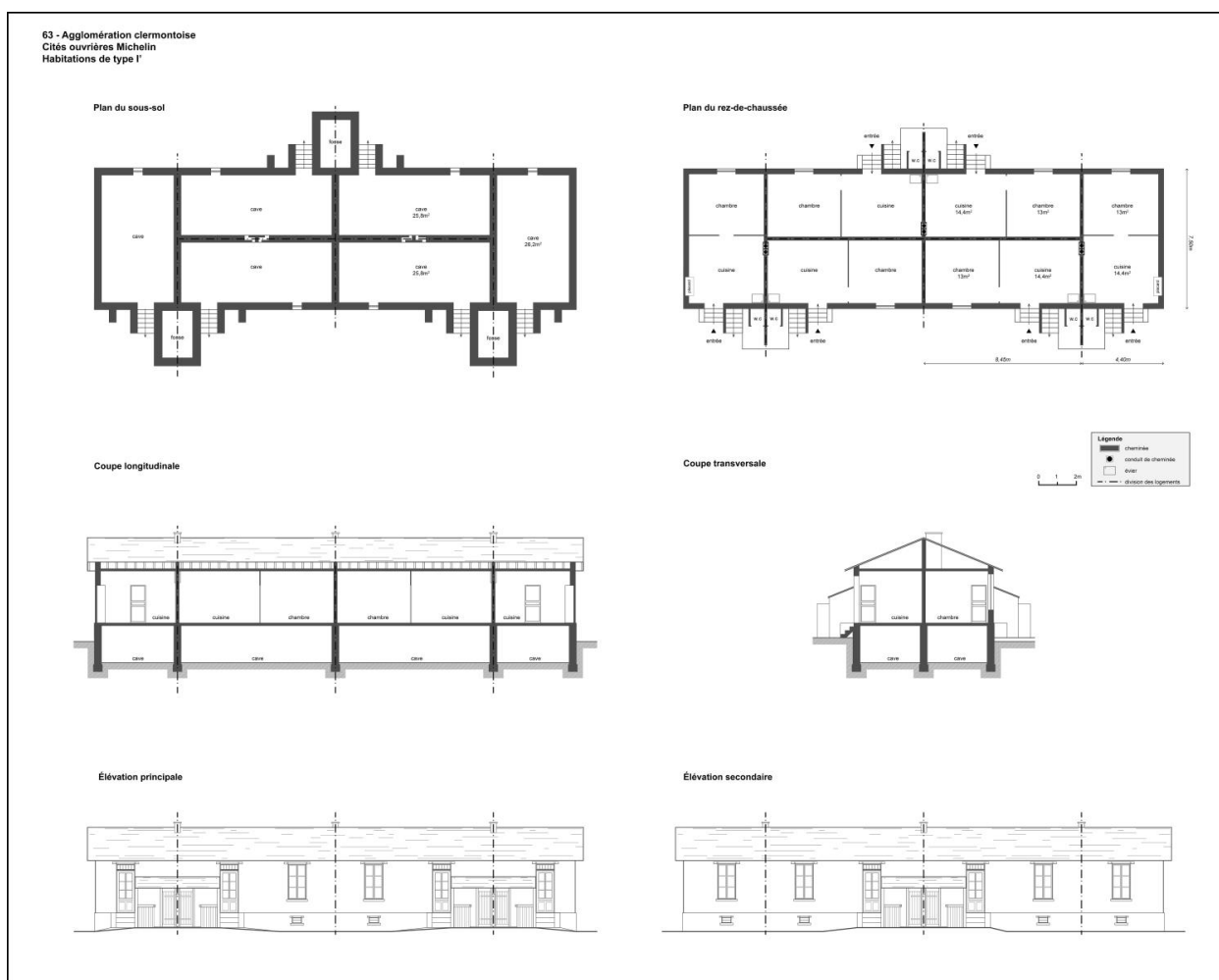
Plan des habitations de type I'.
