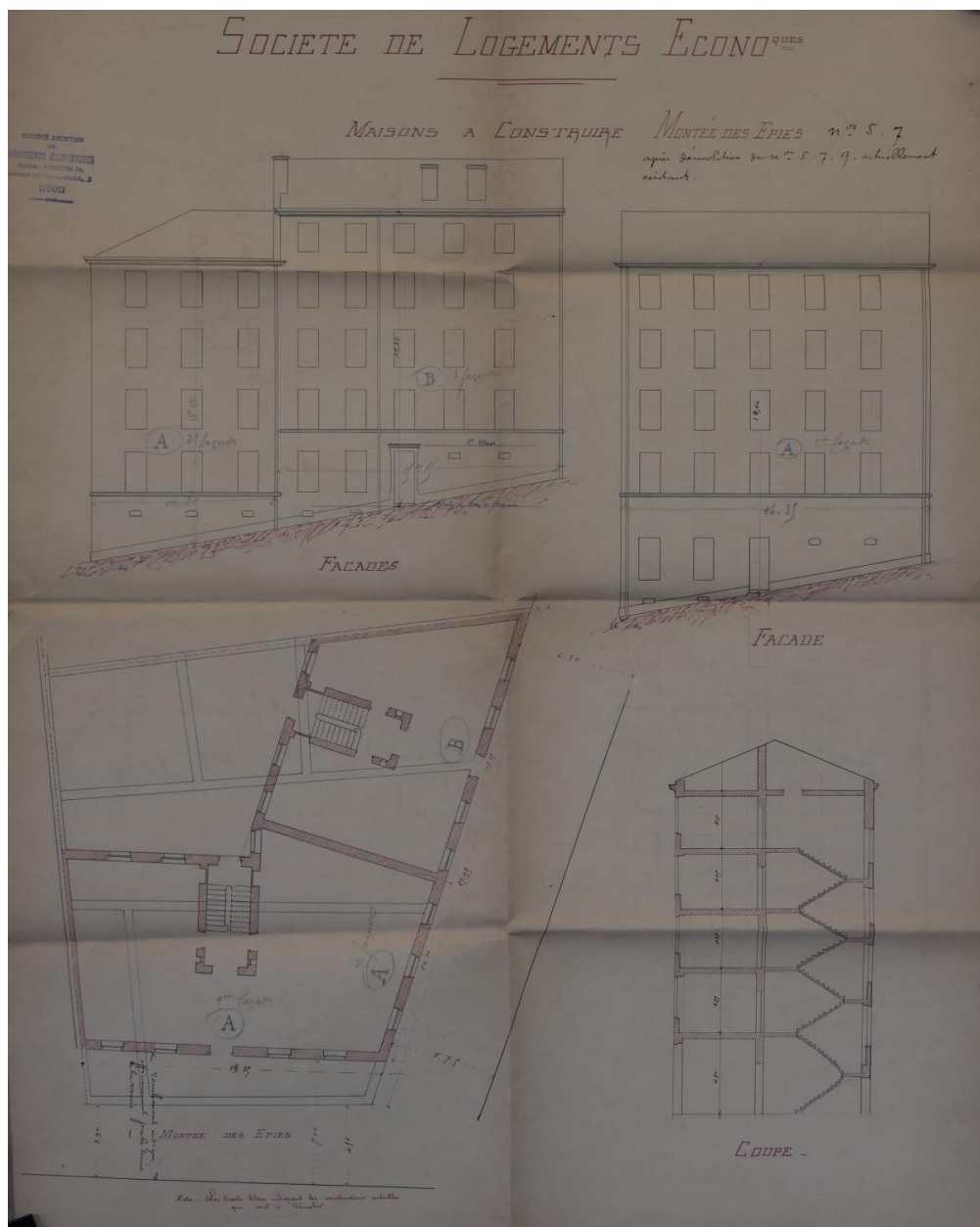
Plans des logements économiques de la Montée des Epies à Saint-Georges en 1890 (ACL 314W56 146)
