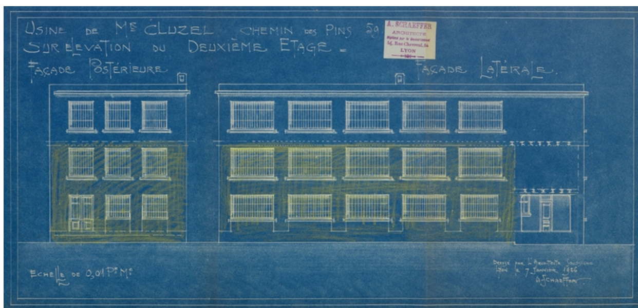
AC Lyon : 344 WP 202 PCA n°0211, élévation façade postérieure de l'usine (surrélévation) de M. Cluzel par M. Schaeffer, 1926
