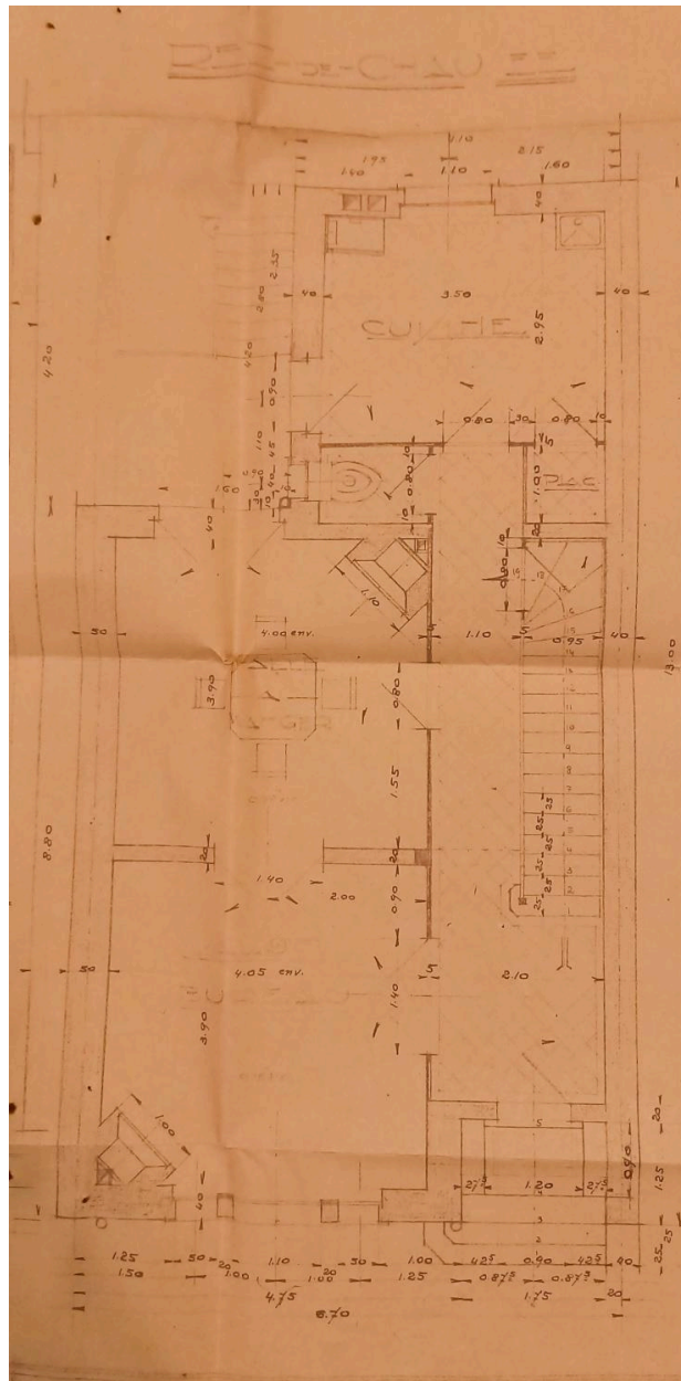
Plan du rez-de-chaussée du 23 boulevard Cote-Blatin
