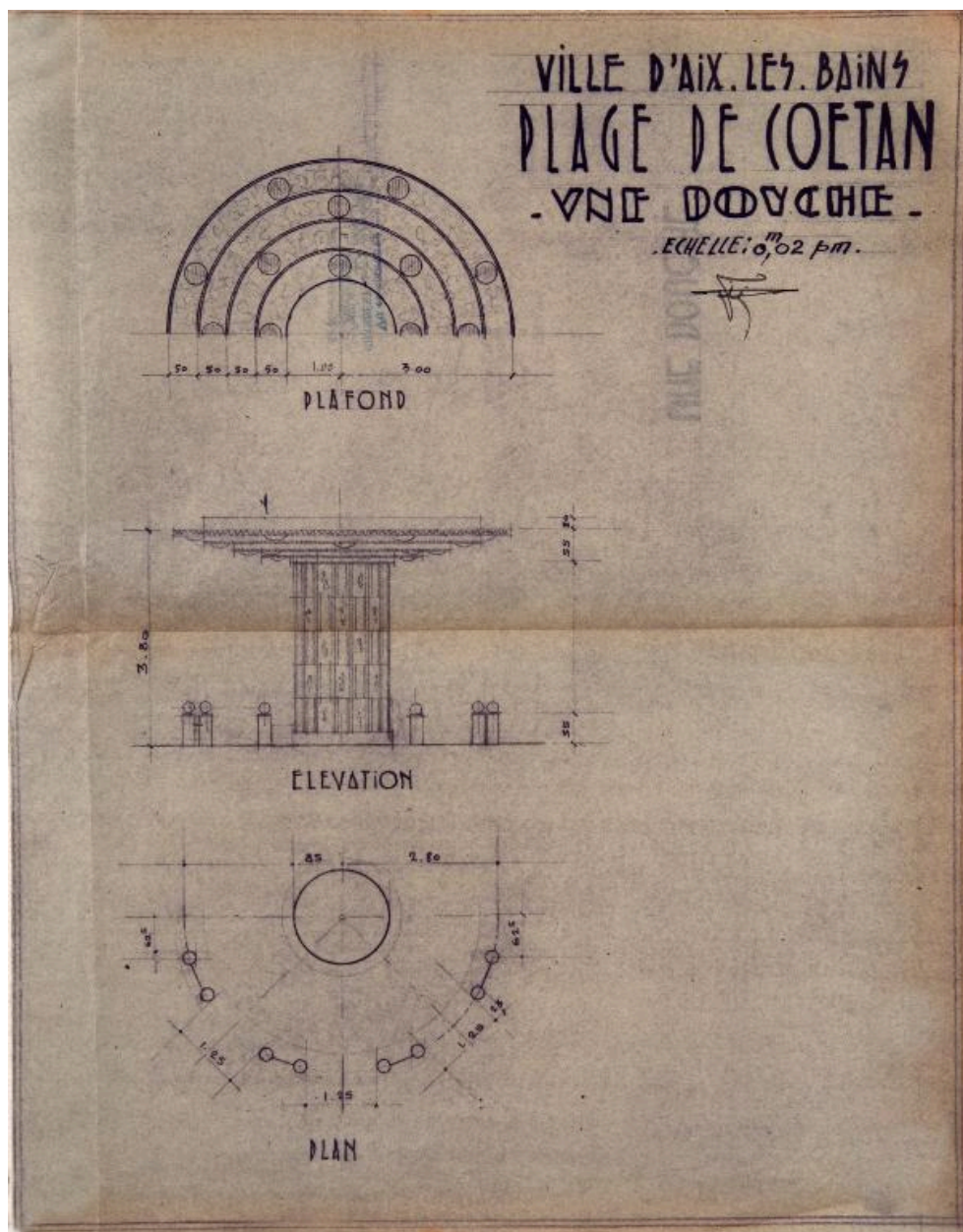
Plan et élévation des douches, 1932
