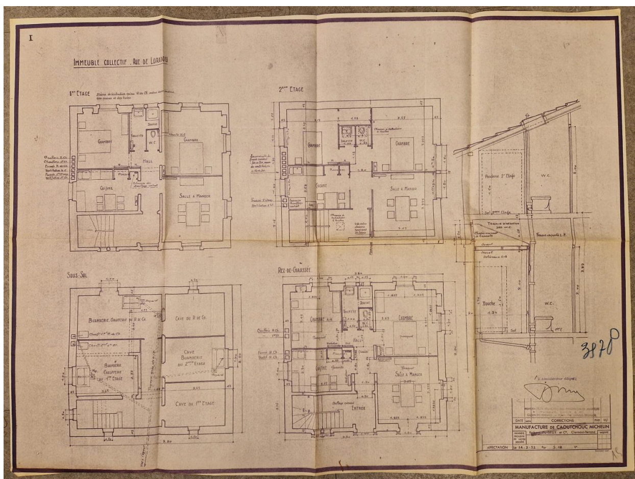
Projet d'immeuble collectif rue de l'Oradou : plans des sous-sol, rez-de-chaussée, 1er et 2e étages, et coupe de détail, 1952.
