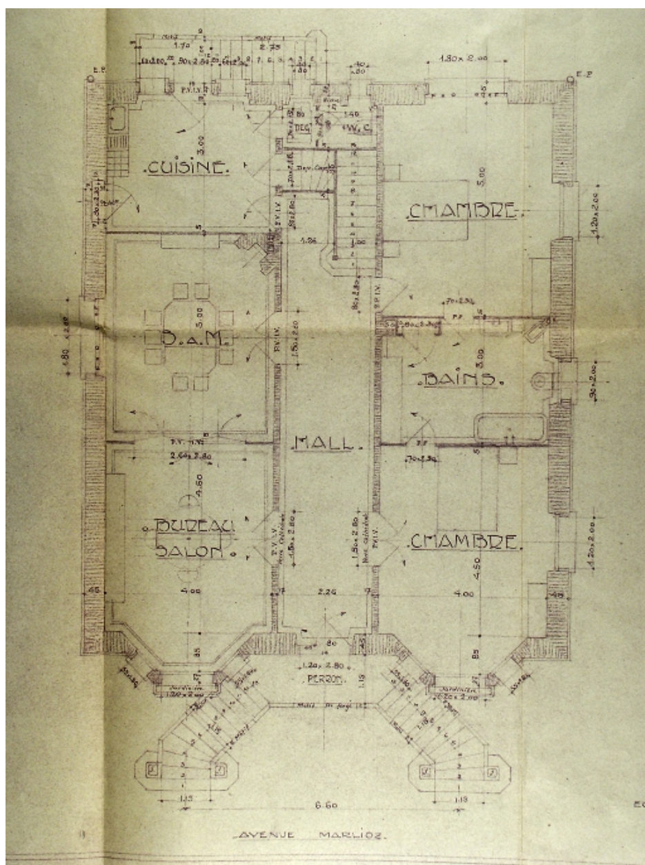
Plan du rez-de-chaussée surélevé
