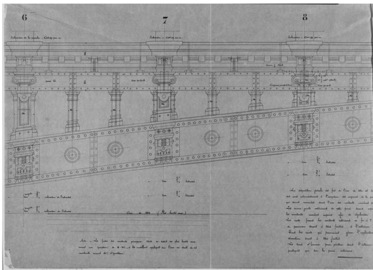
N° 2. Travée centrale de 67 m 40. Détail de l'arc de tête et de sa décoration en fonte entre les montants n° 6 et 13. Paris, Cie de Fives-Lille, 1er avril 1889 (AD Rhône. Cie Fives-Lille. Portefeuille 368 C)
