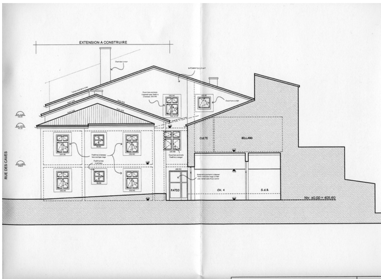
Plan n°6. Façade ouest.
