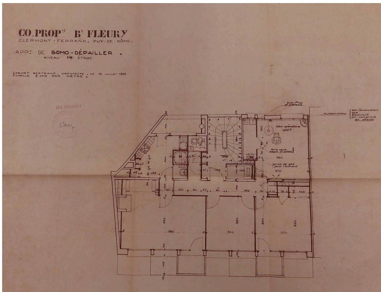
Plan du premier étage (1958)
