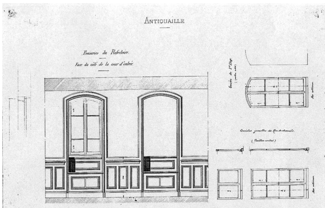
Projet pour la reconstruction des ailes est et sud du cloître, par Paul Pascalon, 1881. 16) Boiserie du réfectoire. Face du côté du cloître
