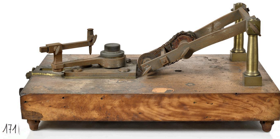
Machine à tailler les engrenages, vue 1
