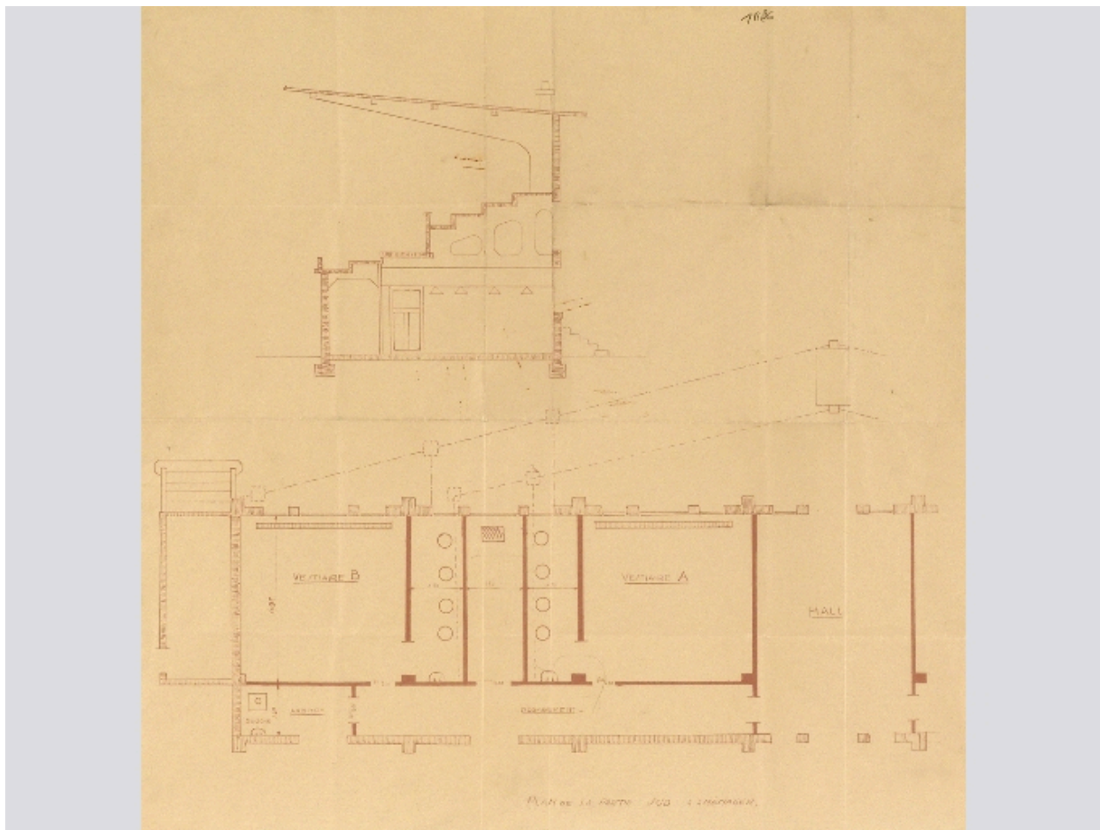
Plan et coupe de la tribune
