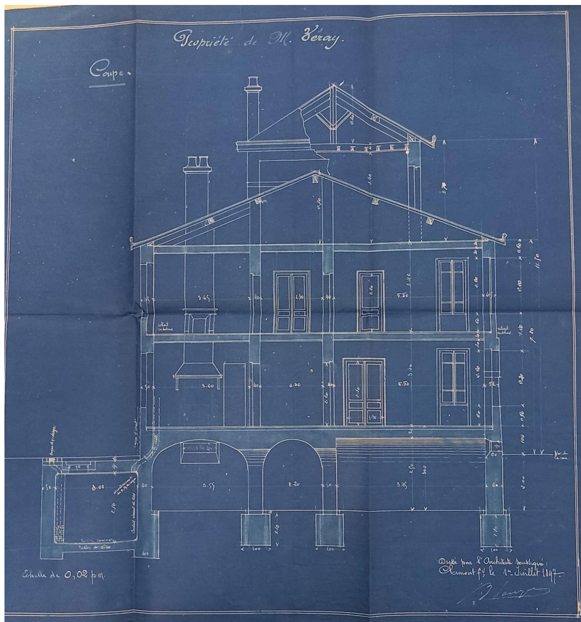
Coupe de la villa, 50 avenue d'Italie
