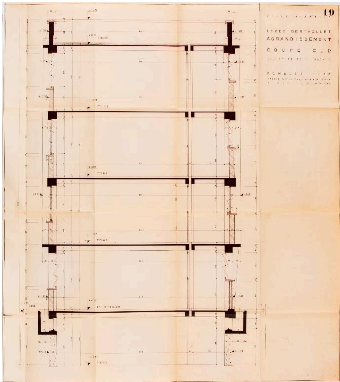
Coupe C-D sur avenue du Petit Brogny, 1963.
