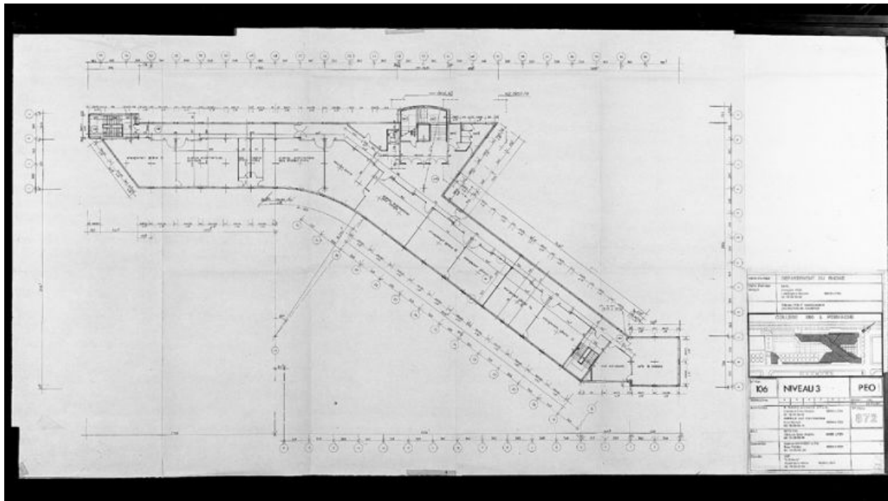
Plan du troisième étage carré
