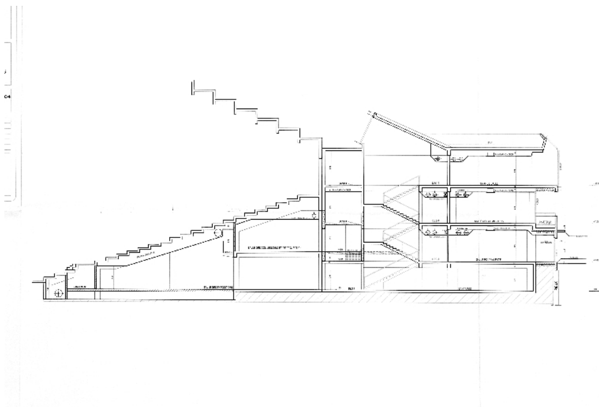
Coupe sur le corps antérieur, vue depuis l'est
