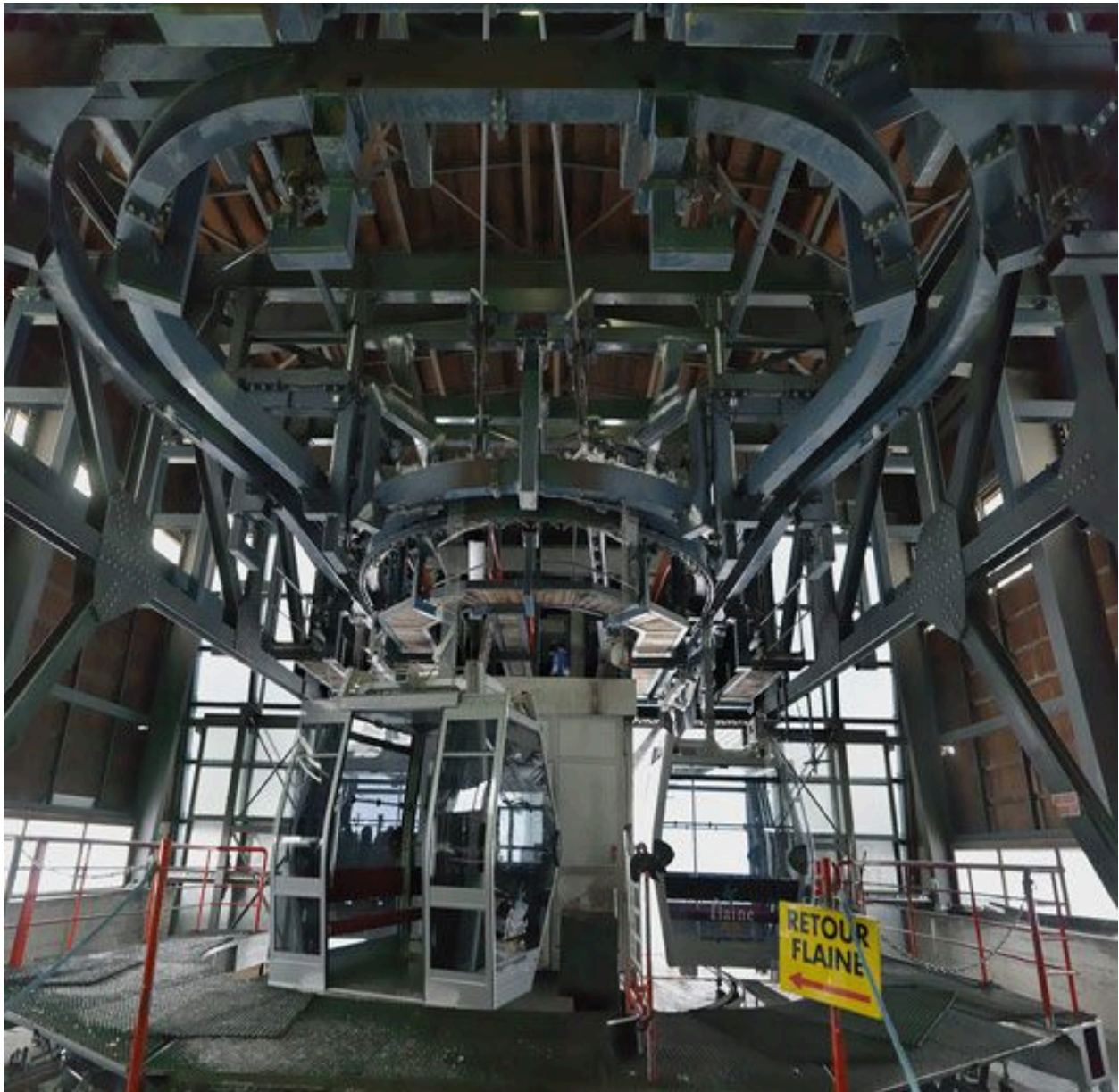
Le mécanisme d'entrainement des cabines de la gare supérieure
