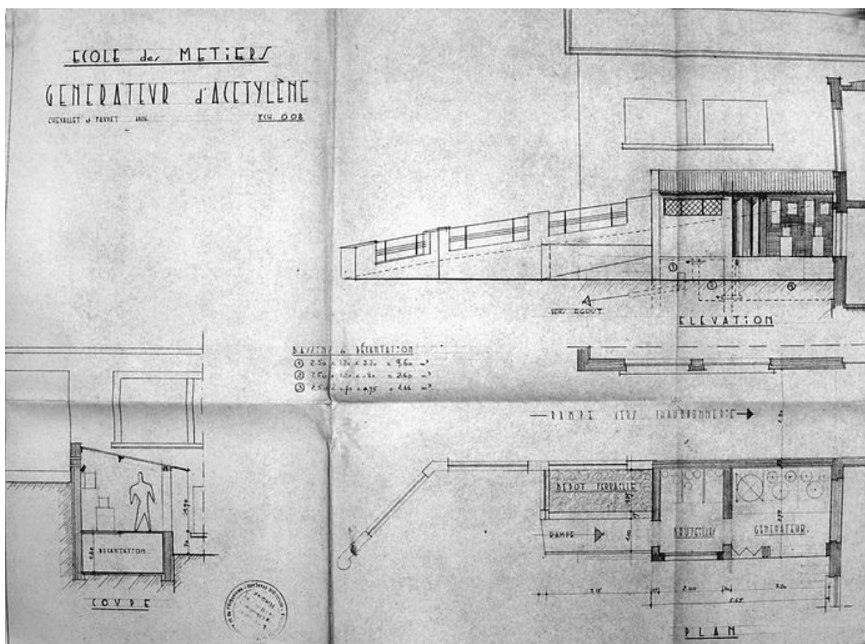
Générateur d'acétylène : coupe, élévation, plan (Chevallet et Fauvet)
