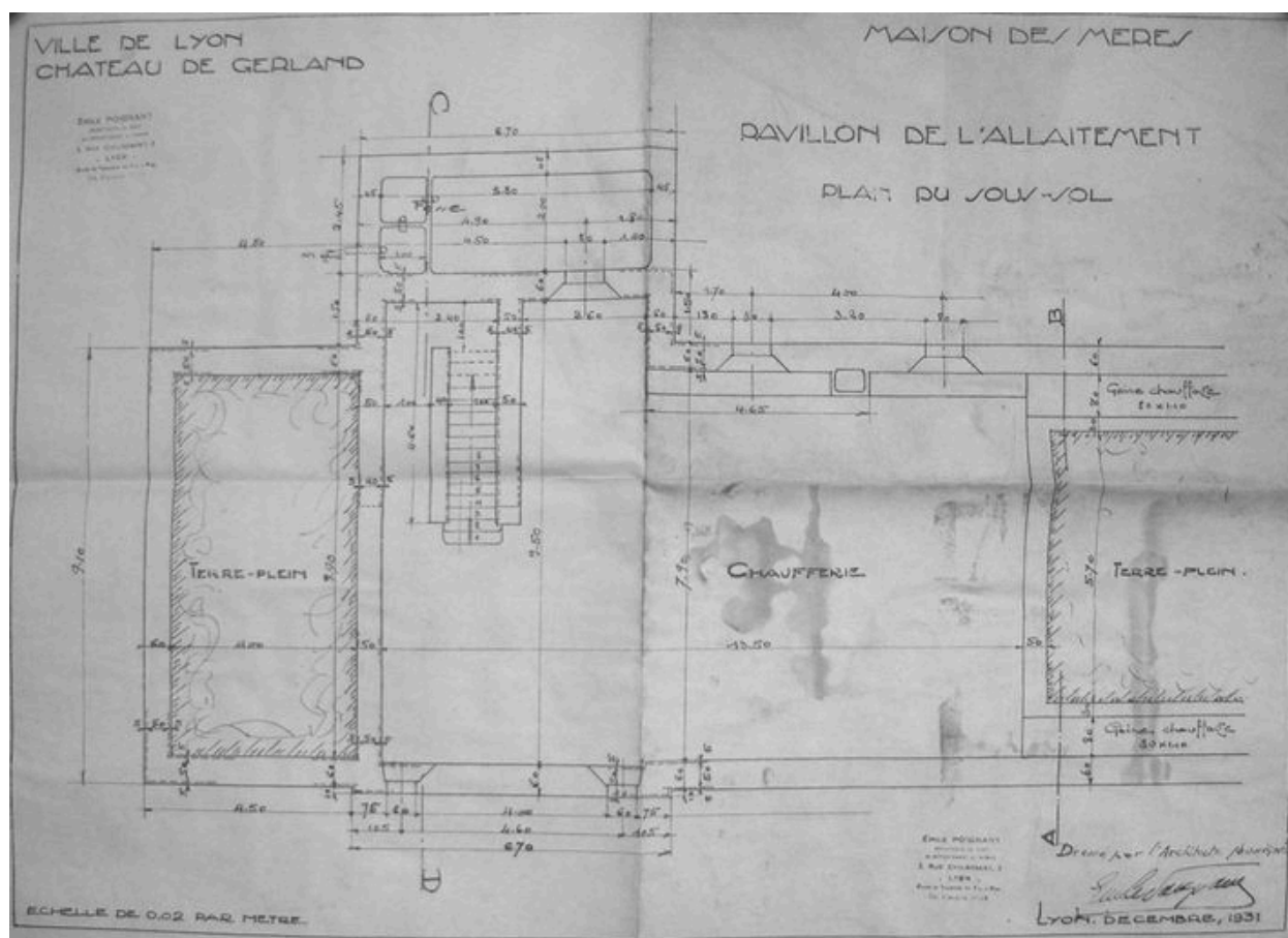
Pavillon de l'allaitement, plan du sous-sol, Emile Poignant architecte, 1931 (AC Lyon 1741 W 5)
