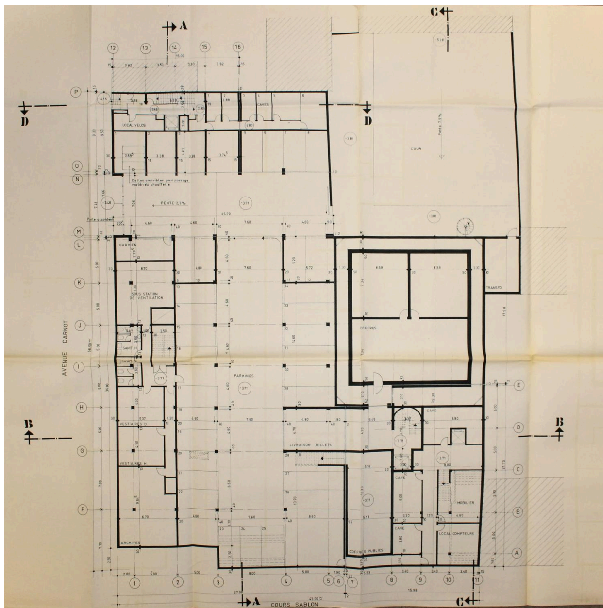
Clermont-Ferrand, succursale de la Banque de France, plan du sous-sol semi-enterré, 1971, agence ATEA Lagneau-Weil-Dimitrijevic (Archives municipales de Clermont-Ferrand, 2001 W 296).
